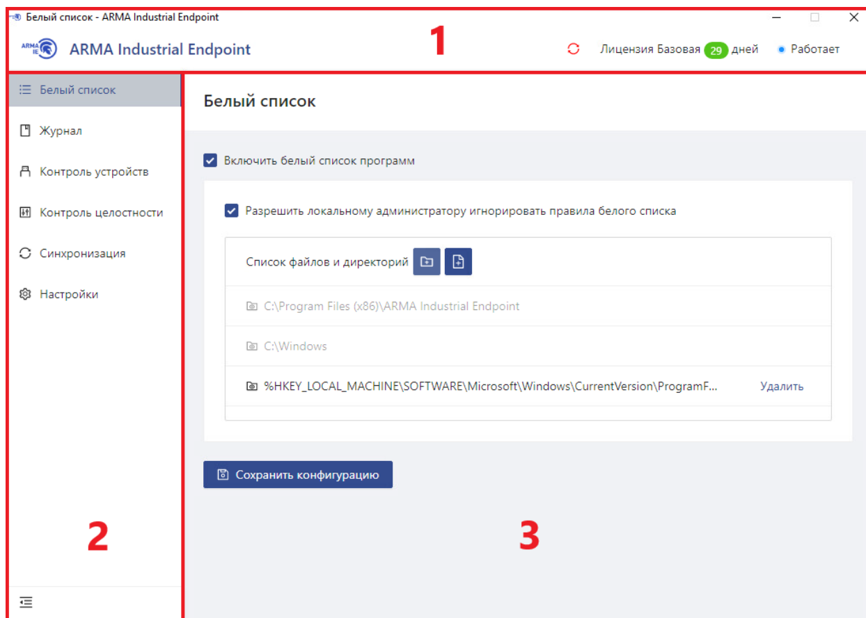
Рисунок – Локальный графический интерфейс ARMA IE
