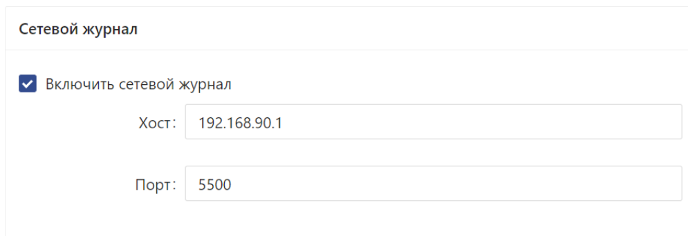
Рисунок – Блок настроек «Сетевой журнал».
