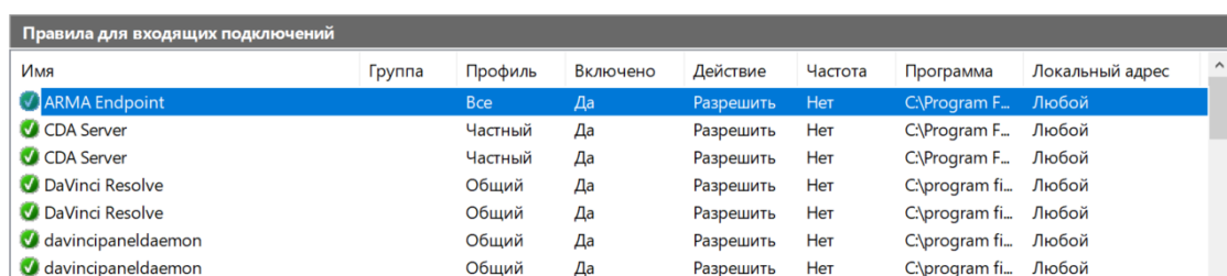
Рисунок – Правило МЭ
