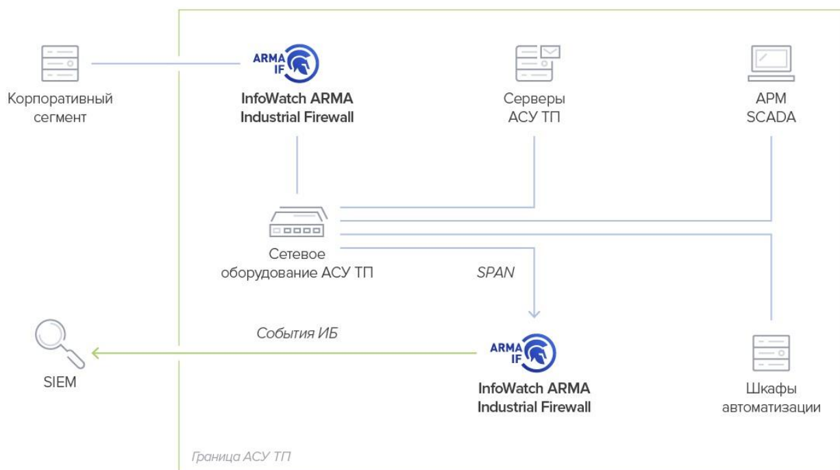
Рисунок 9 – Применение для мониторинга внутри АСУ ТП
