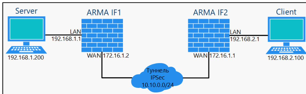
Рисунок 211 – Схема стенда для настройки IPsec в режиме «сеть» - «сеть»
