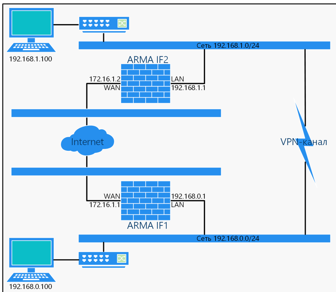
Рисунок 191 – Схема стенда для настройки OpenVPN в режиме «сеть - сеть»
