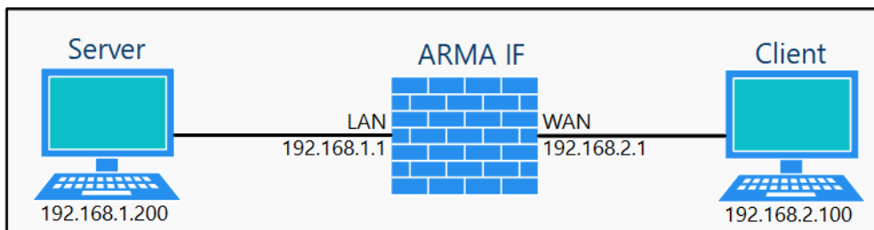
Рисунок 59 – Схема стенда для проверки срабатывания правил COB
