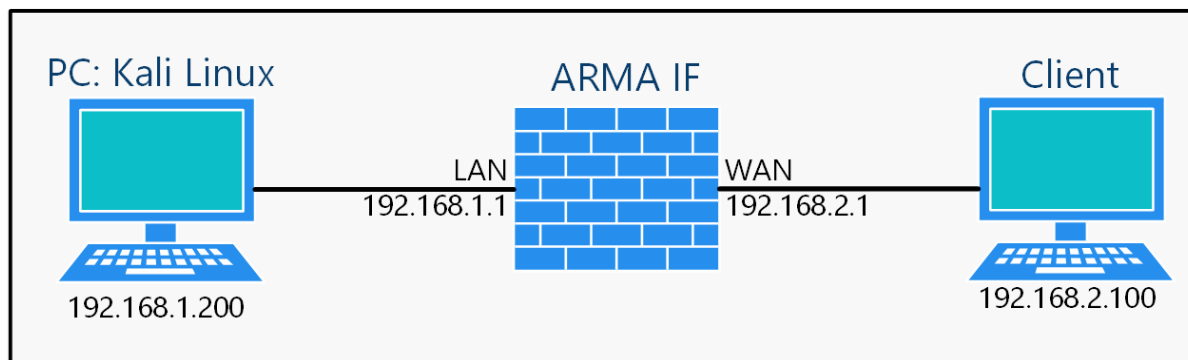
Рисунок 65 – Схема стенда для проверки срабатывания пользовательского правила на DOS- атаку
