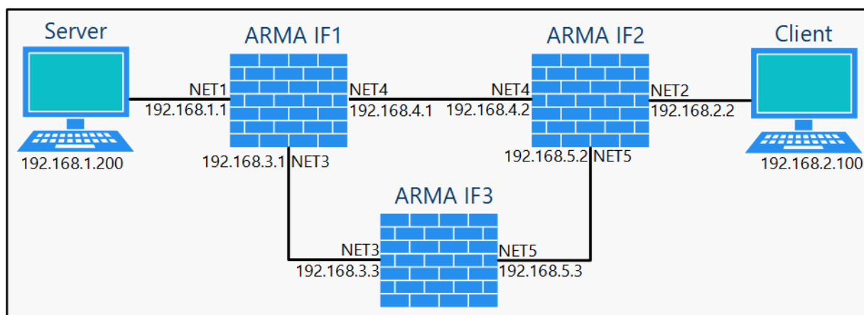
Рисунок 116 – Схема стенда для настройки динамической маршрутизации
