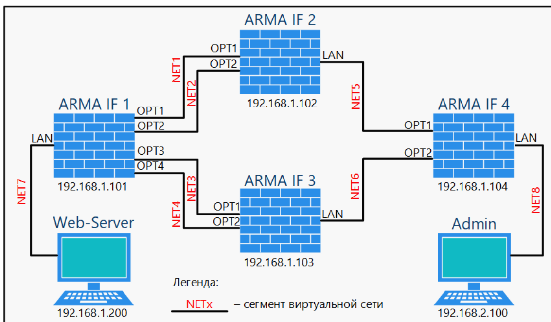
Рисунок 162 – Стенд для проверки RSTP
