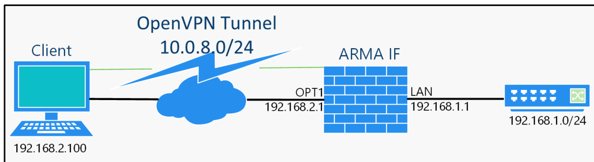
Рисунок 194 – Схема стенда для настройки OpenVPN в режиме «клиент - сеть»
