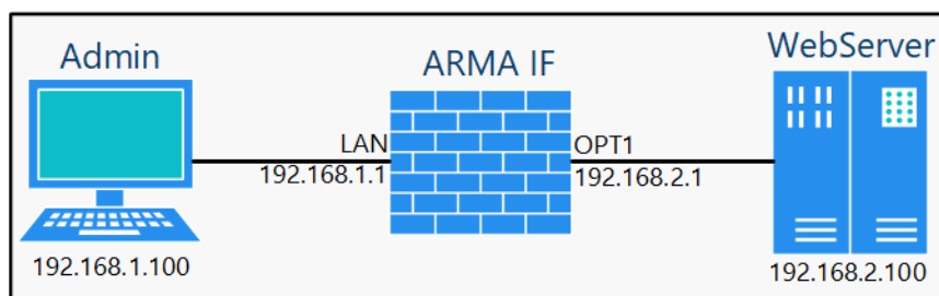
Рисунок 289 – Схема стенда для проверки функции захвата пакетов
