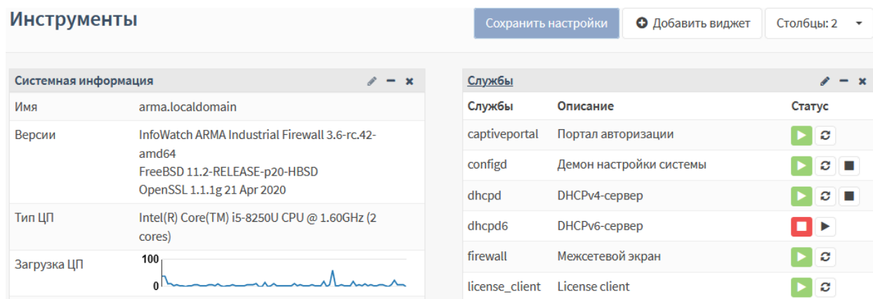
Рисунок 275 – Панель виджетов
