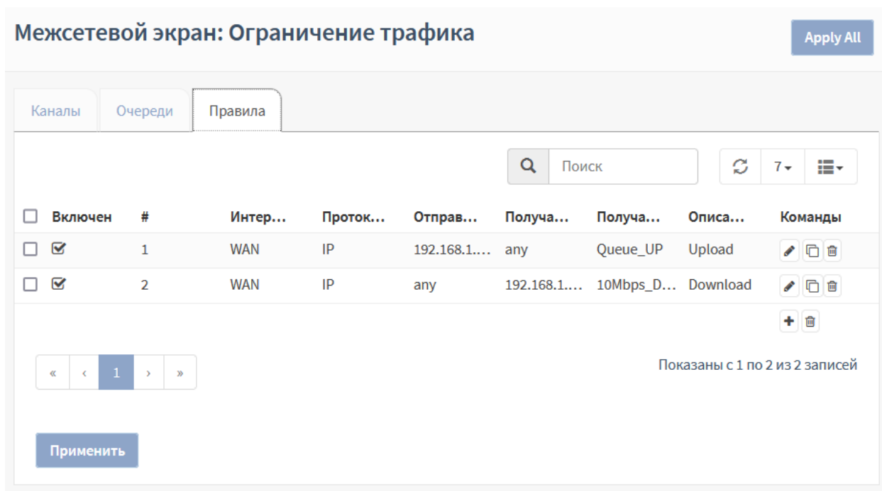
Рисунок 44 – Список правил
