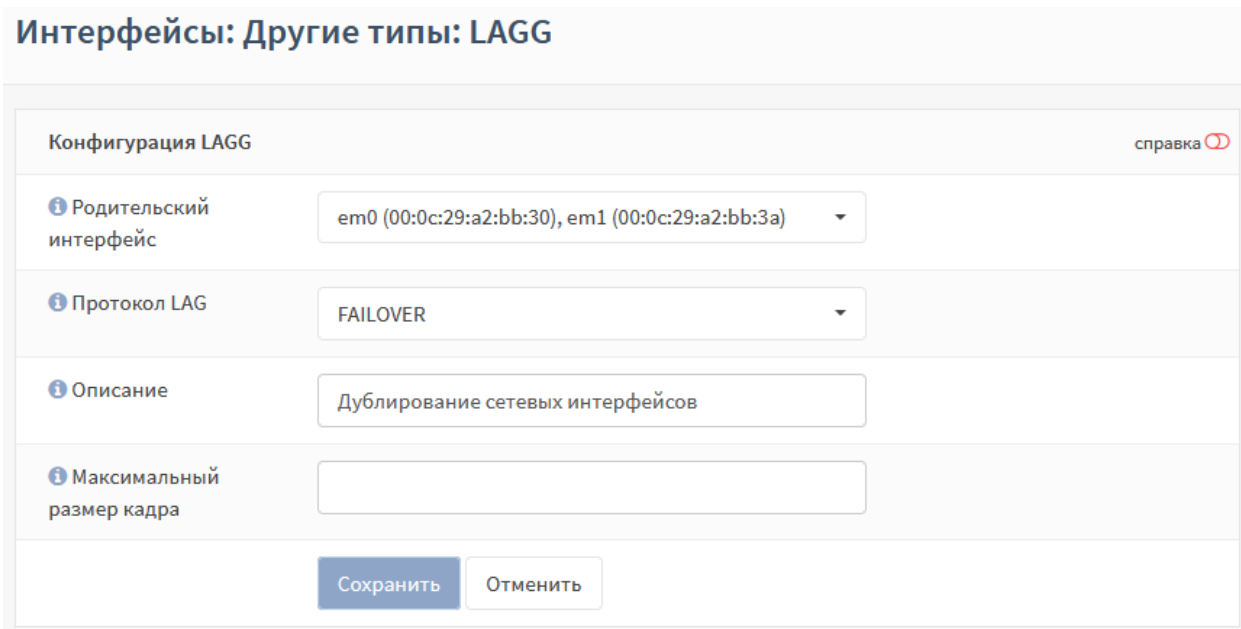
Рисунок 151 – Конфигурация LAGG
