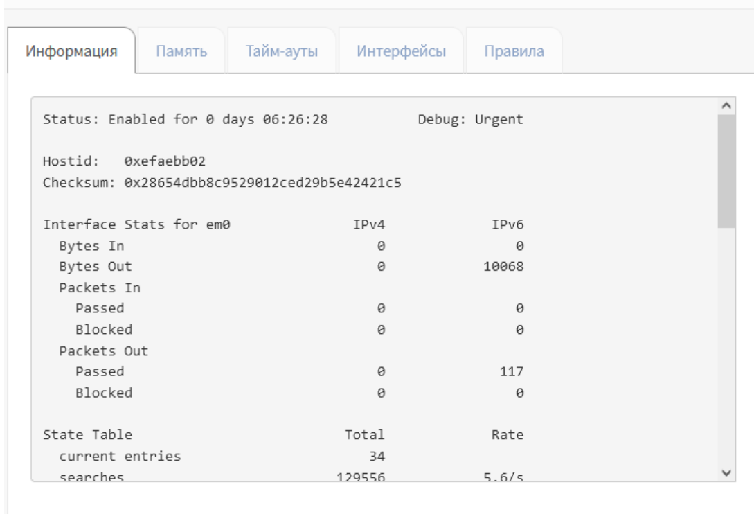
Рисунок 280 – Диагностика pfInfo
