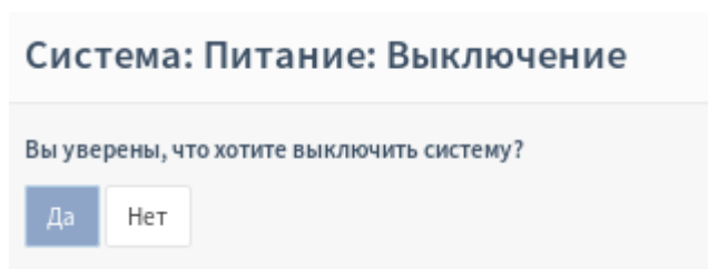
Рисунок 326 – Выключение системы
