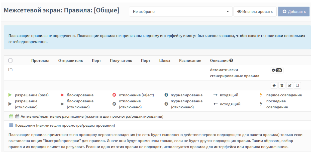
Рисунок 6 – Подраздел «Общие»
