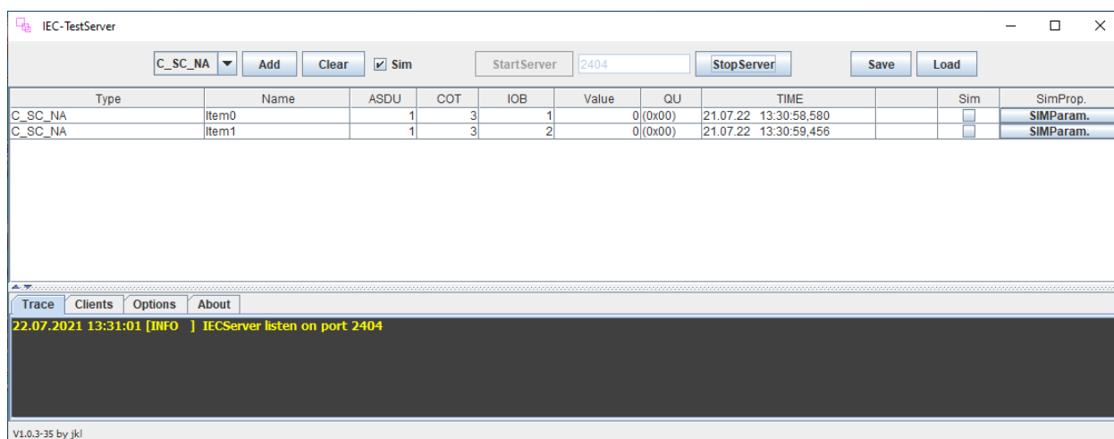
Рисунок 71 – Запуск IECServer
