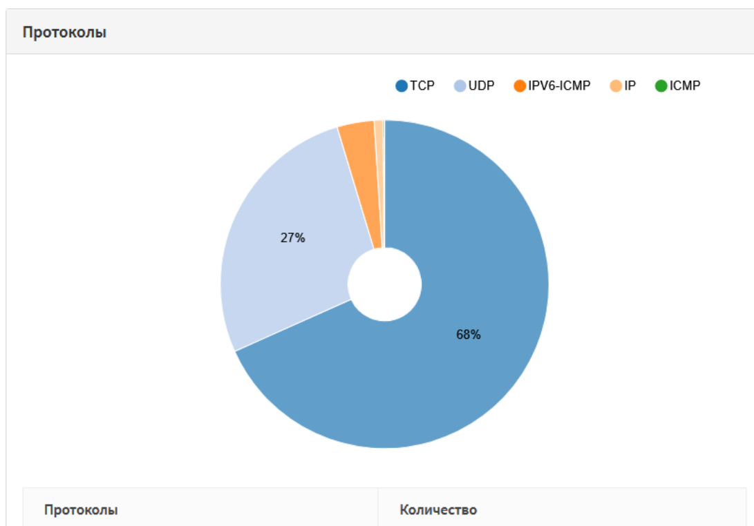
Рисунок 300 – Протоколы
