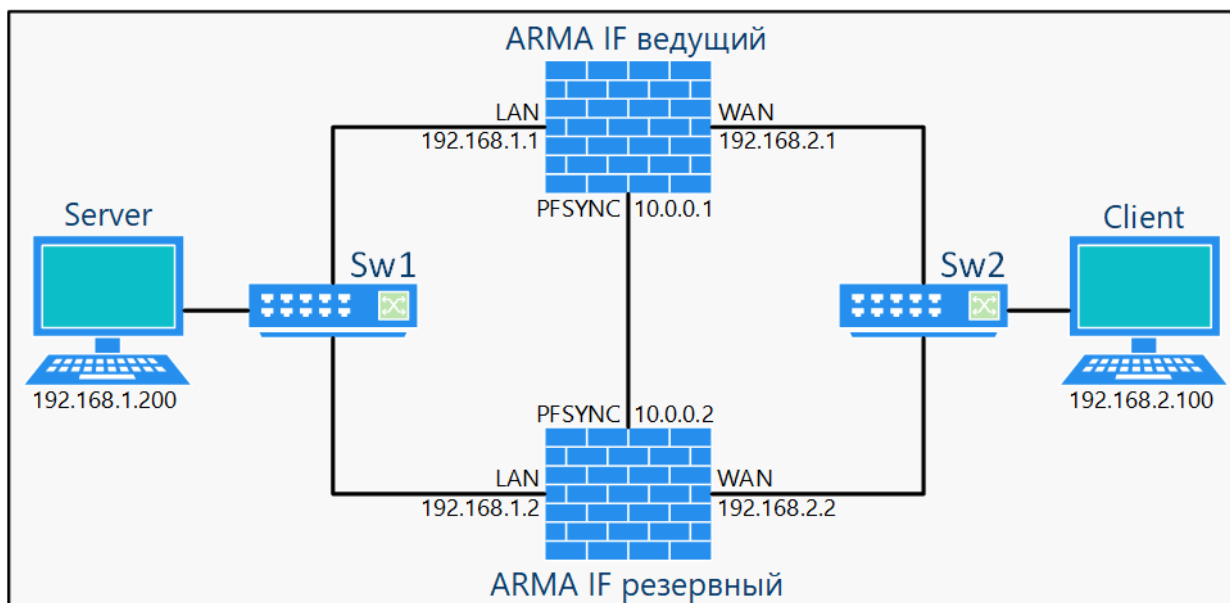
Рисунок 47 – Схема стенда для настройки режима отказоустойчивого кластера
