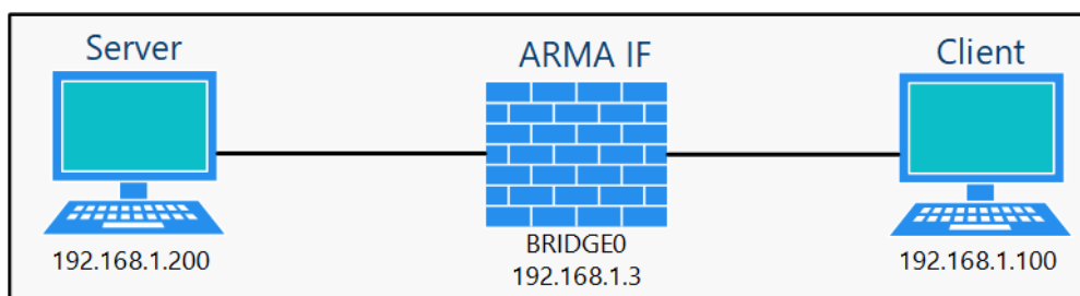
Рисунок 158 – Схема стенда для настройки сетевого моста
