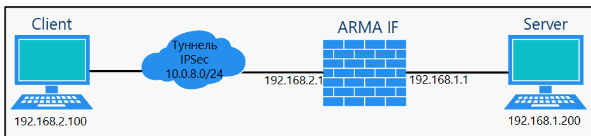
Рисунок 197 – Схема стенда для настройки IPsec в режиме «узел» - «сеть»
