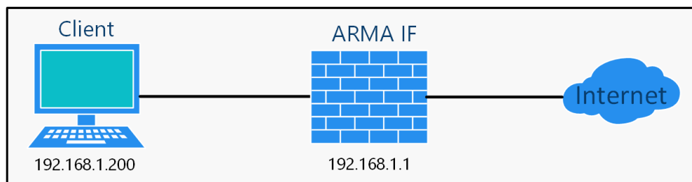
Рисунок 269 – Схема стенда настройки Dnsmasq
