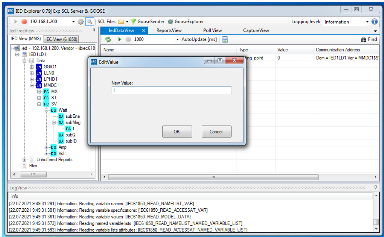
Рисунок 90 – Запись значения
