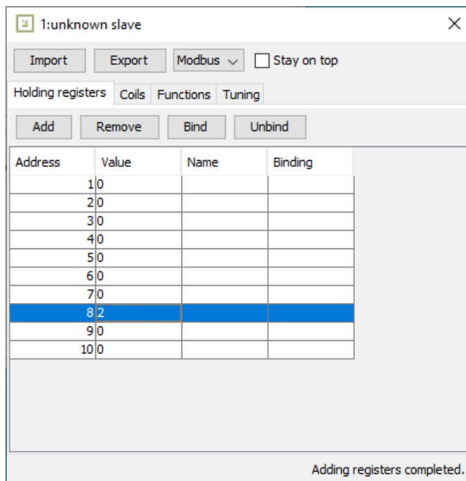
Рисунок 69 – Запись данных
