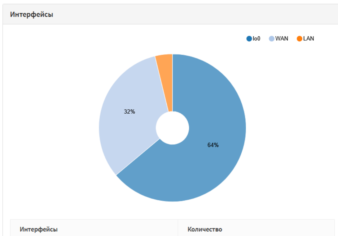
Рисунок 299 – Интерфейсы
