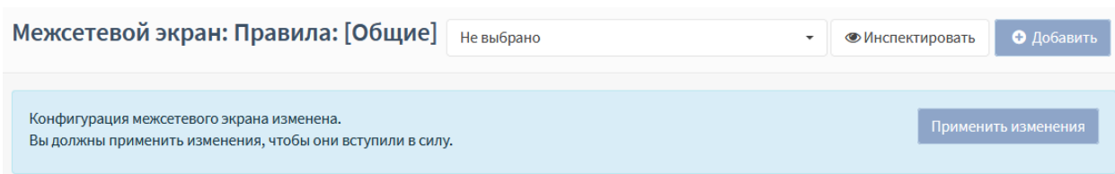
Рисунок 8 – Принятие изменений
