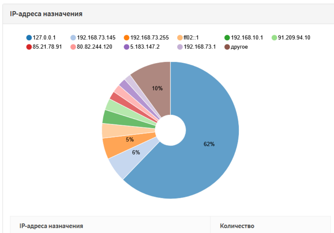
Рисунок 302 – IP-адреса назначения
