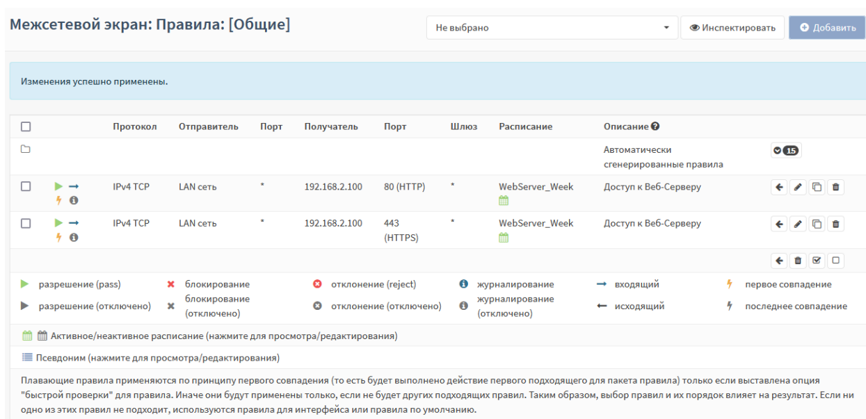
Рисунок 3 – Список правил
