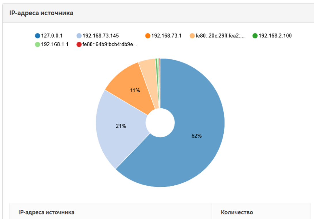
Рисунок 301 – IP-адреса источника
