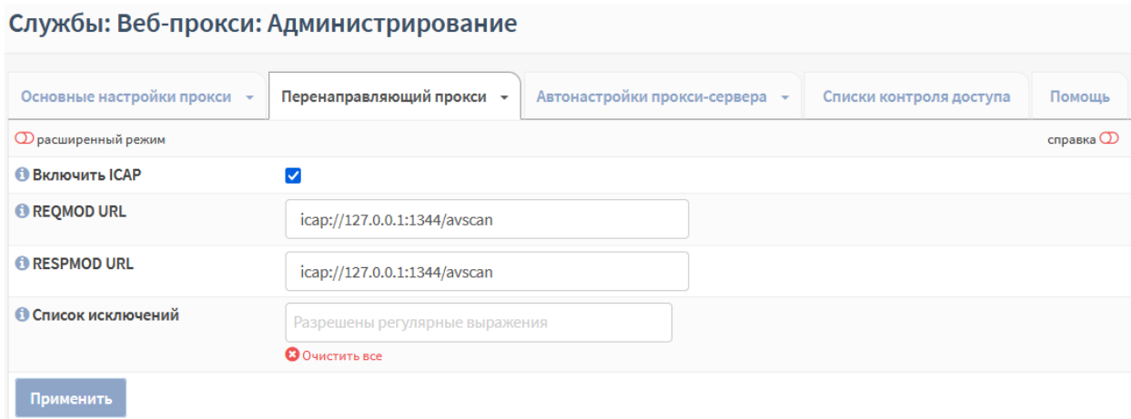
Рисунок 260 – Настройка ICAP
