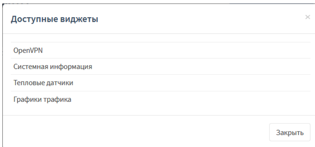
Рисунок 276 – Добавление виджетов
