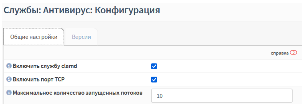
Рисунок 264 – Включение антивируса
