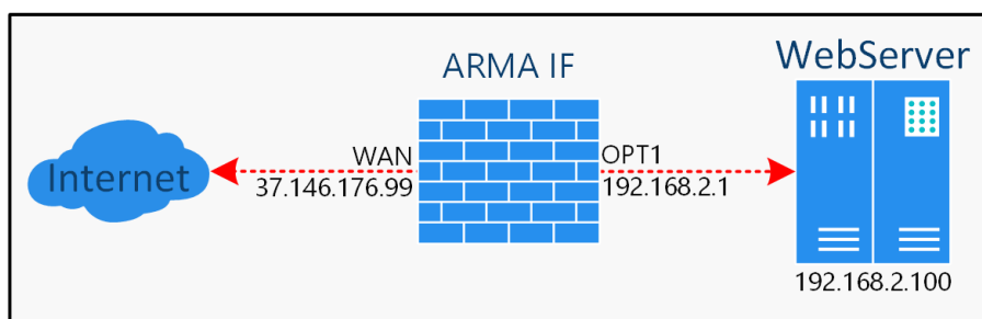
Рисунок 29 – NAT «Один-к-одному»
