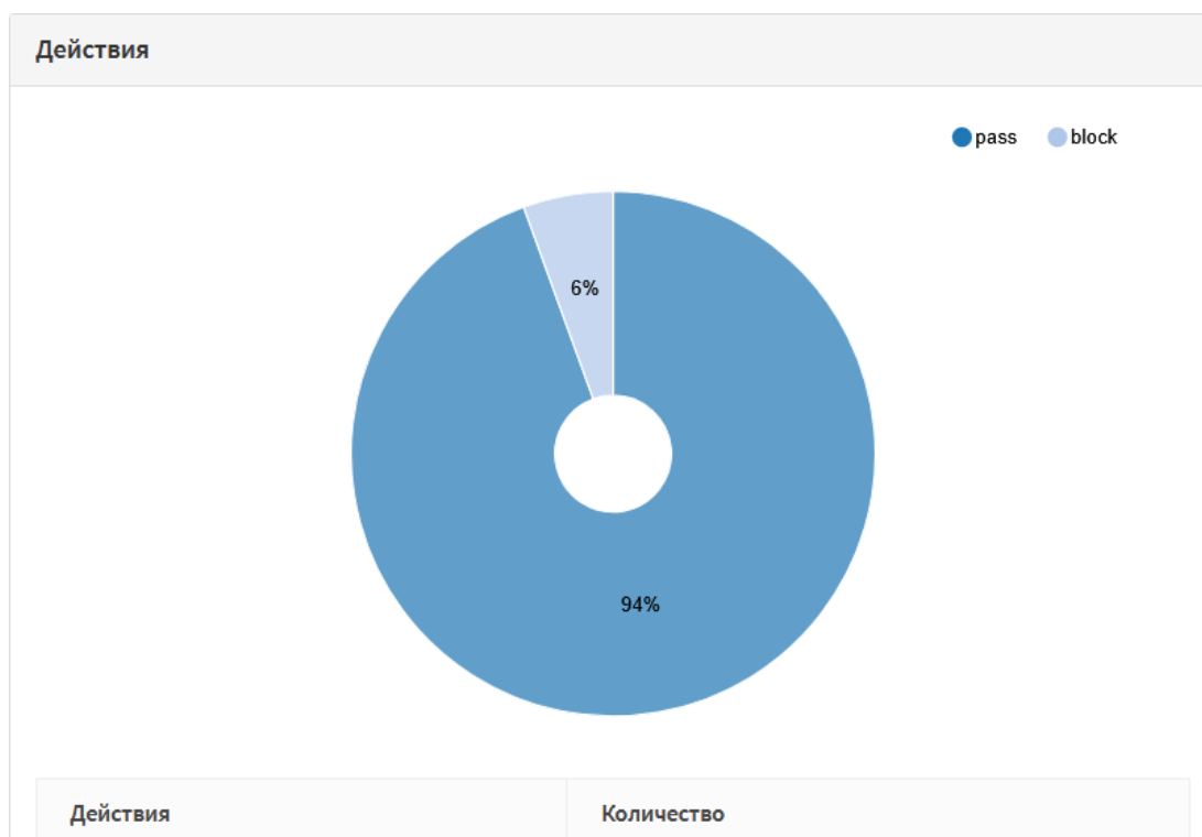
Рисунок 298 – Действия
