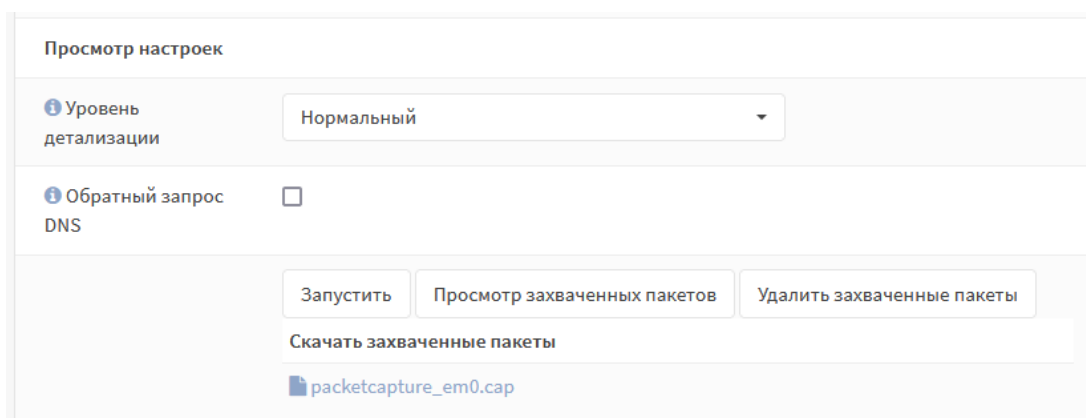
Рисунок 291 – Дамп трафика
