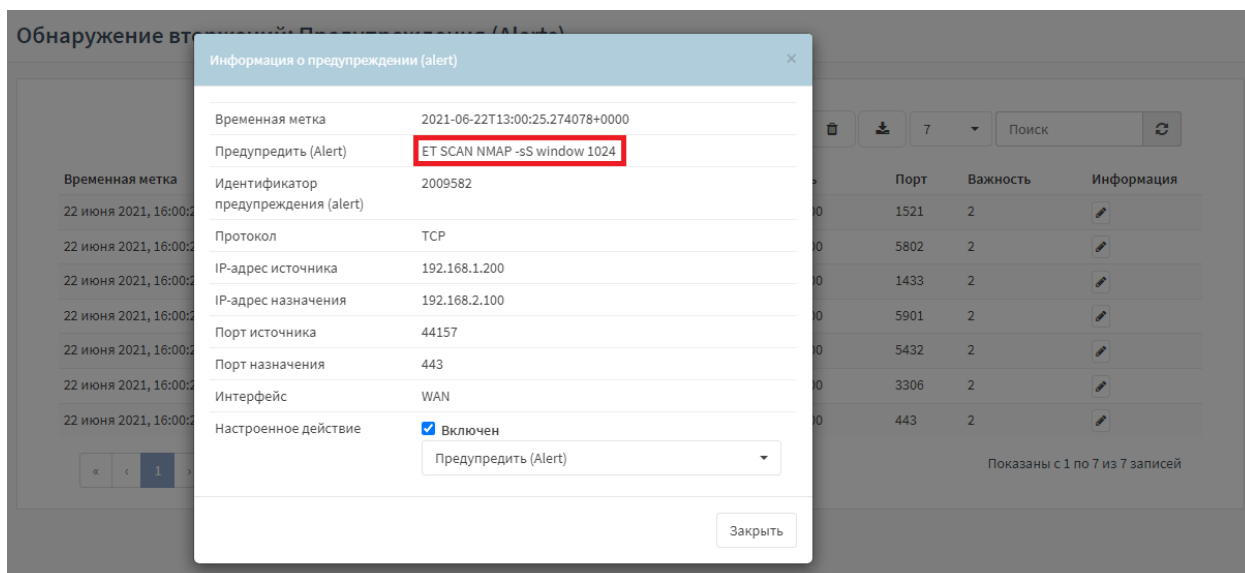
Рисунок 61 – Результаты сканирования
