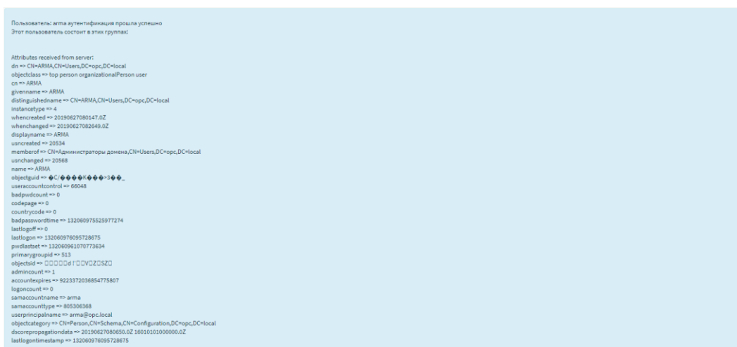
Рисунок 236 – Успешная аутентификация
