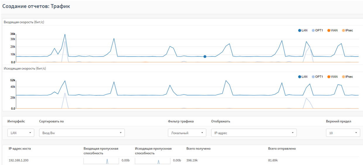
Рисунок 324 – Трафик
