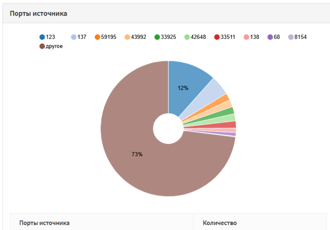
Рисунок 303 – Порты источника
