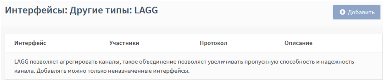
Рисунок 150 – Подраздел LAGG
