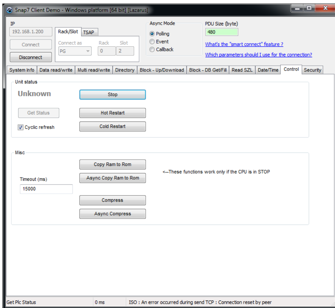
Рисунок 78 – Отключение контроллера
