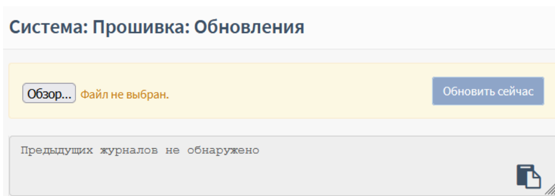
Рисунок 254 – Обновление системы
