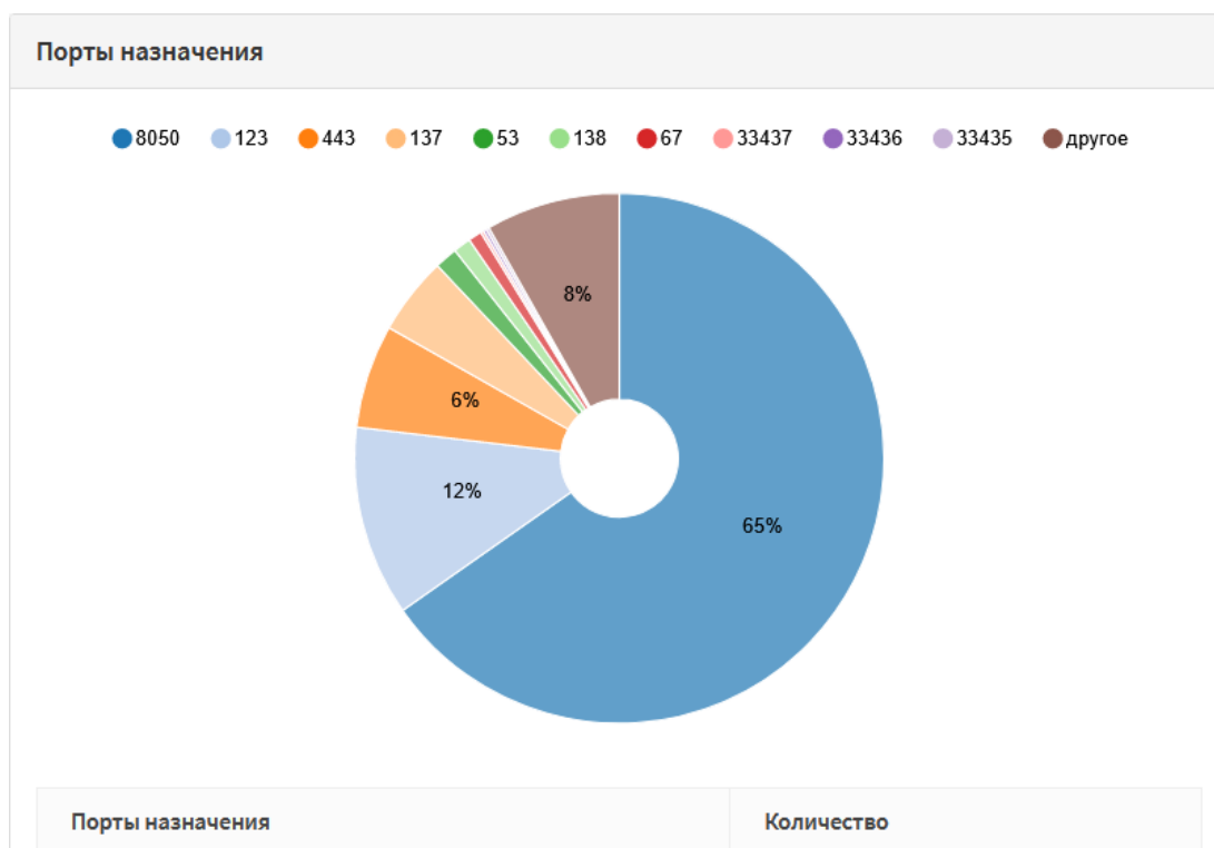
Рисунок 304 – Порты назначения
