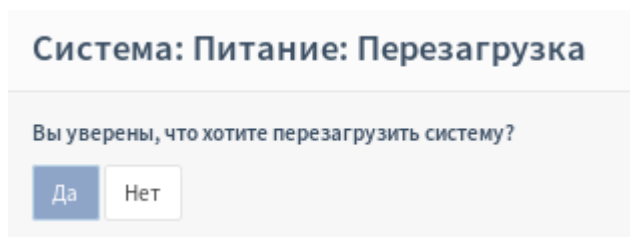
Рисунок 325 – Перезагрузка системы
