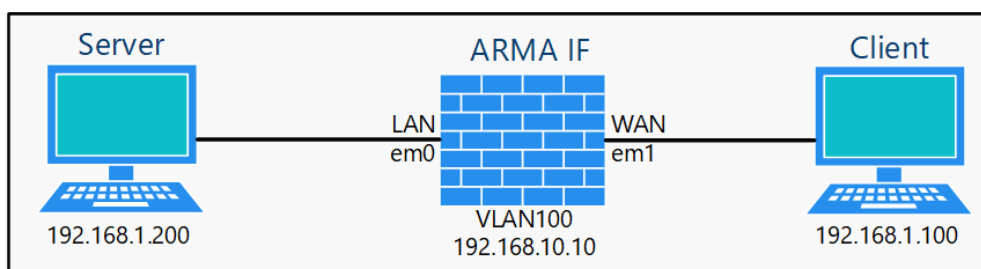
Рисунок 172 – Схема стенда для настройки VLAN
